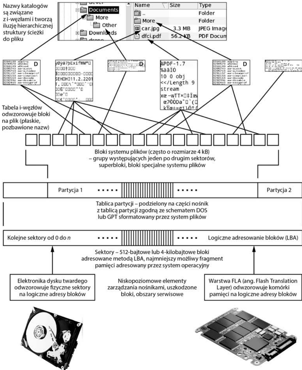
Rysunek 3.2. Abstrakcja systemu plików. (Jest to uproszczony schemat, który nie obejmuje grup bloków, redundancji, skalowalności i innych specjalnych funkcjonalności)
