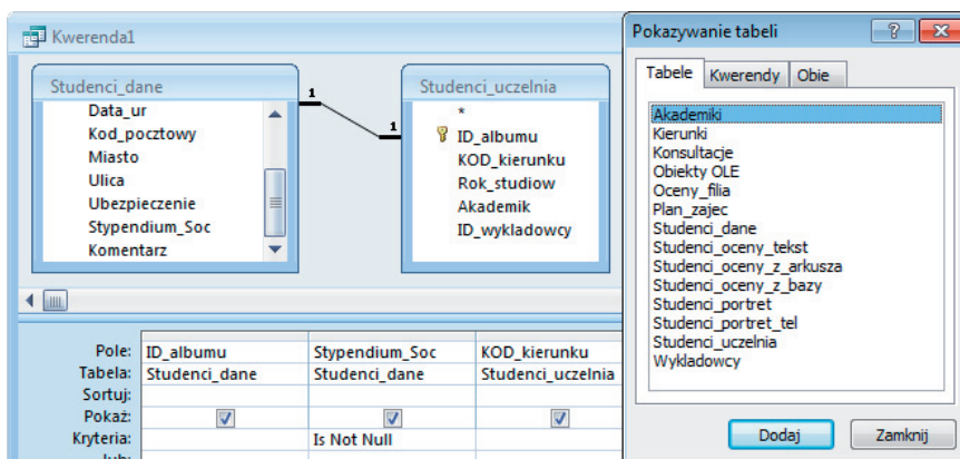
Rysunek 2.34. Okno wyboru tabel do projektu kwerendy
